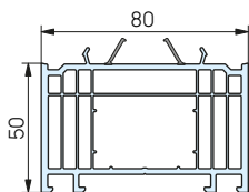
875050 Розширювач 50
