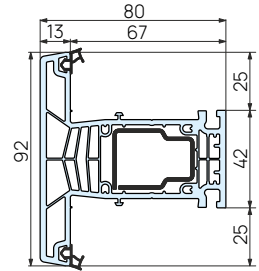
873010 Імпост MD
