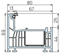
871010 Рама MD
