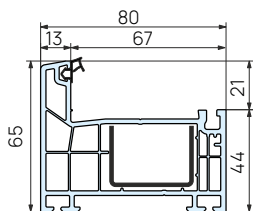
871005 Рама AD
