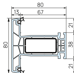
873005 Імпост AD
