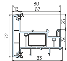
873020 Штульп
