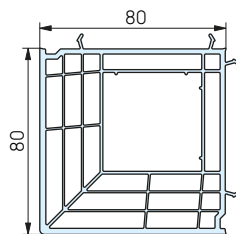
875120 З'єднувач кутовий 90°
