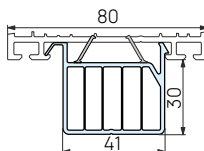
876030 Профіль підставочний 30
